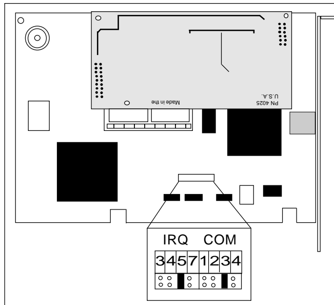
The BOCA M144DI MODEM
