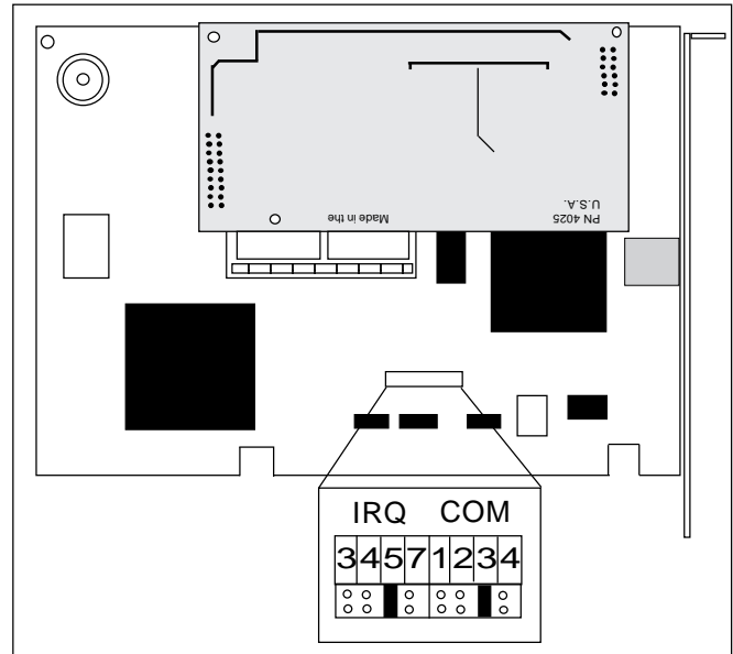
The BOCA M144NI MODEM
