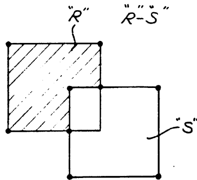
(d) DIFFERENCE
