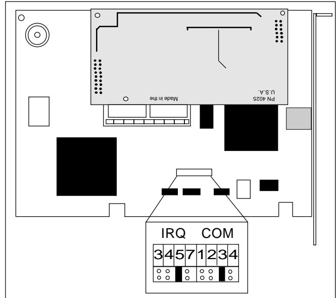
The BOCA M144GI MODEM
